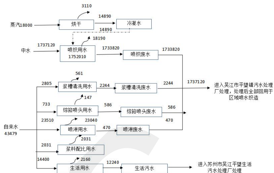
图2-1改建前水平衡图 t/a
