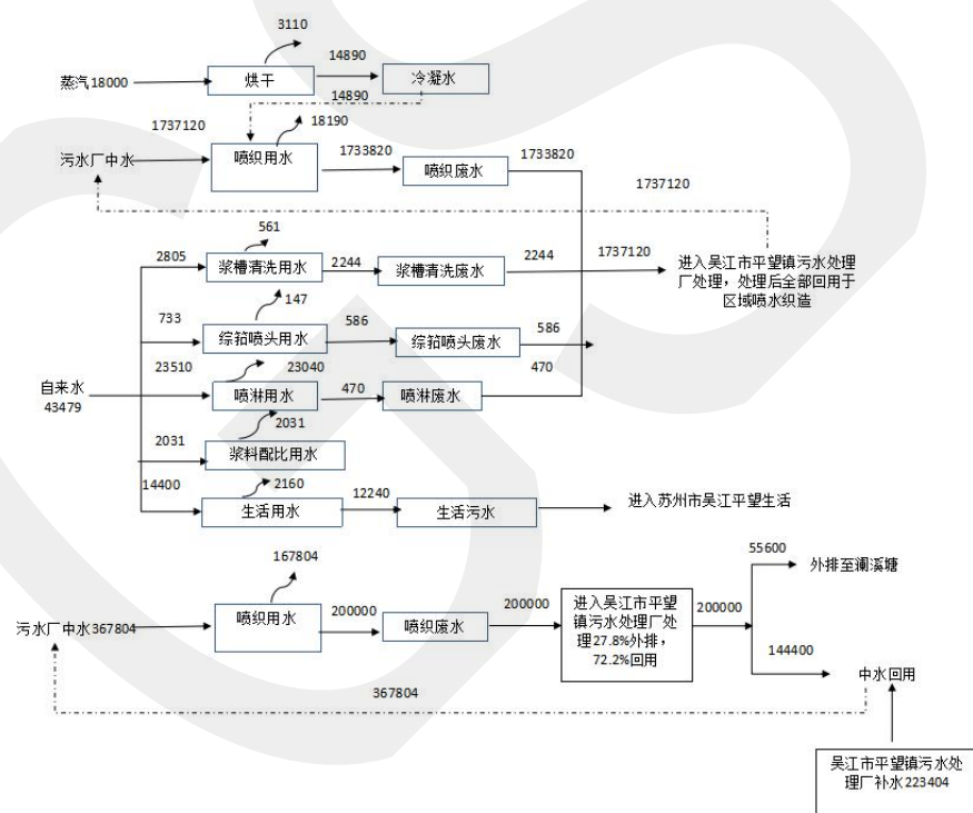
图2-1改建前水平衡图 t/a
