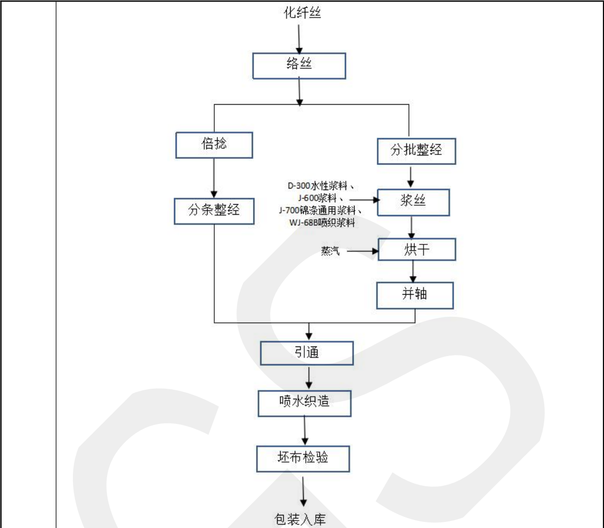
图 2-4 现有项目生产及产污环节示意图
