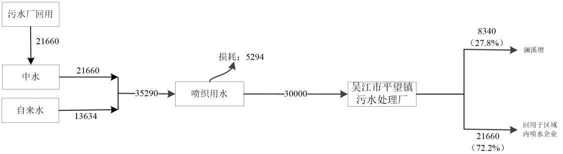
图2-2技改前苏州璟腾纺织有限公司水平衡图 t/a
