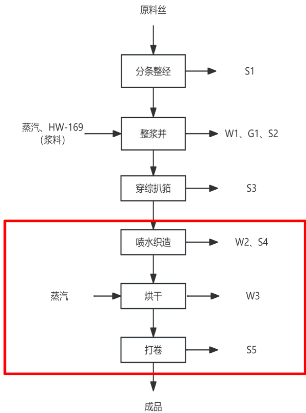
图 2-4 生产工艺流程及产污环节示意图
