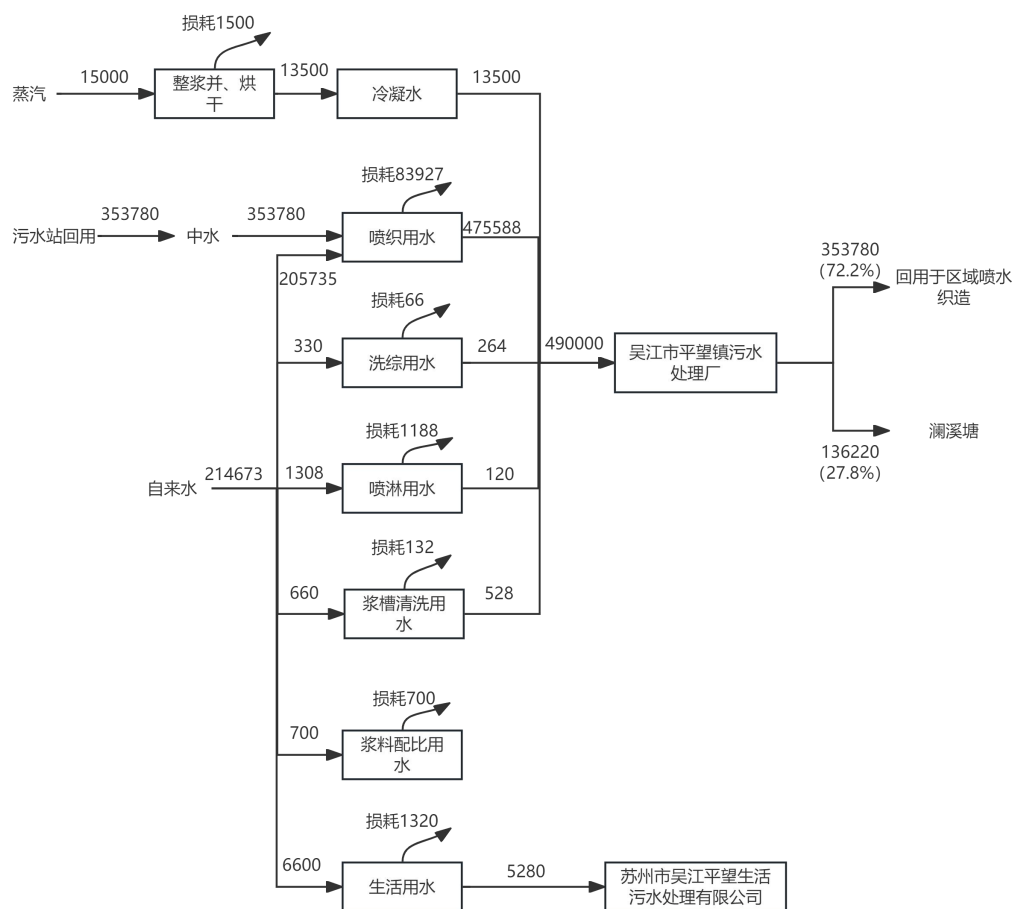
图2-9技改后水平衡图 t/a
