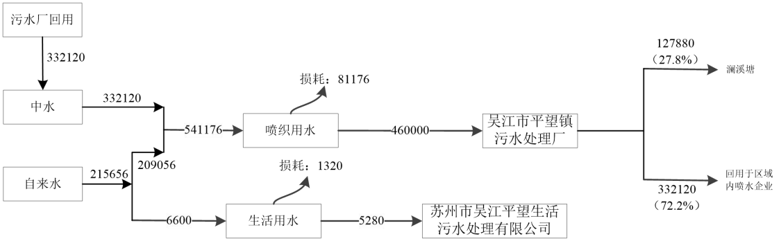
图2-1技改前吴江中晖织造有限公司水平衡图 t/a
