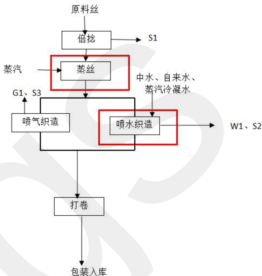
图 2-4 生产工艺流程及产污环节示意图
