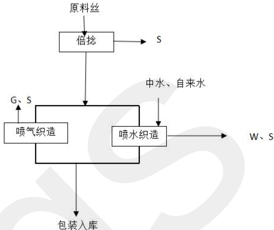
图 2-5 现有项目生产及产污环节示意图
