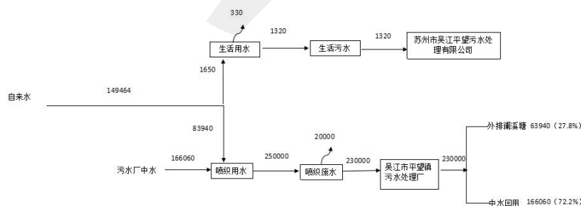
图2-1技改前吴江市展宏纺织有限公司水平衡图 t/a
