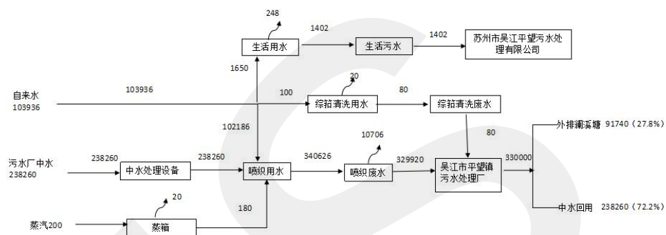
图2-3技改后吴江市展宏纺织有限公司水平衡图 t/a
