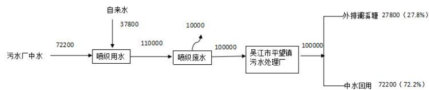
图2-2技改前吴江市弘联织造有限公司水平衡图 t/a
