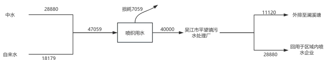
图2-3技改前吴江市锦美来纺织有限公司水平衡图 t/a
