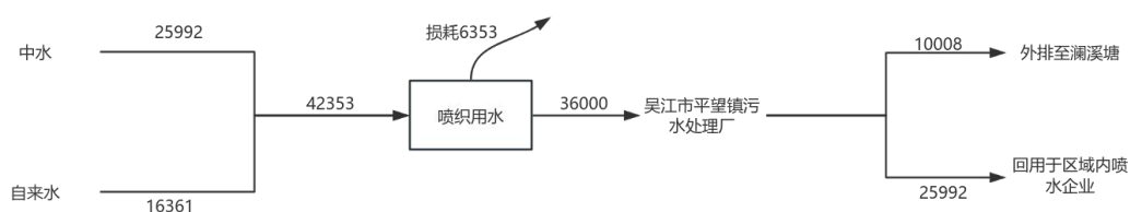
图2-4技改前吴江市帅佳纺织有限公司水平衡图 t/a
