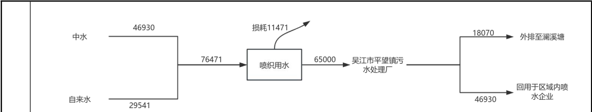
图2-5技改前吴江市常顺纺织有限公司水平衡图 t/a
