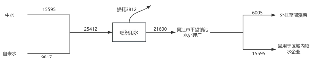
图2-2技改前苏州祥允丰纺织有限公司水平衡图 t/a
