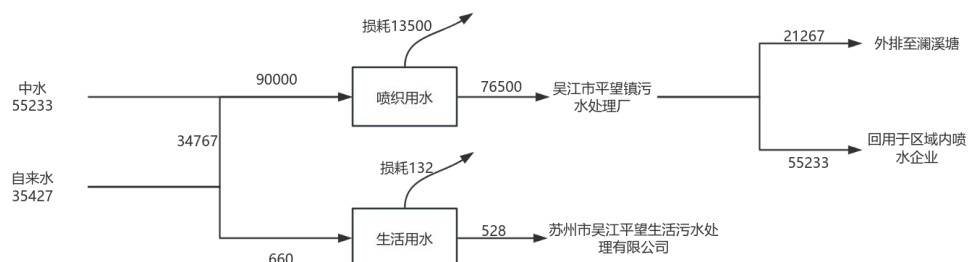
图2-1技改前苏州云舜达纺织有限公司水平衡图 t/a
