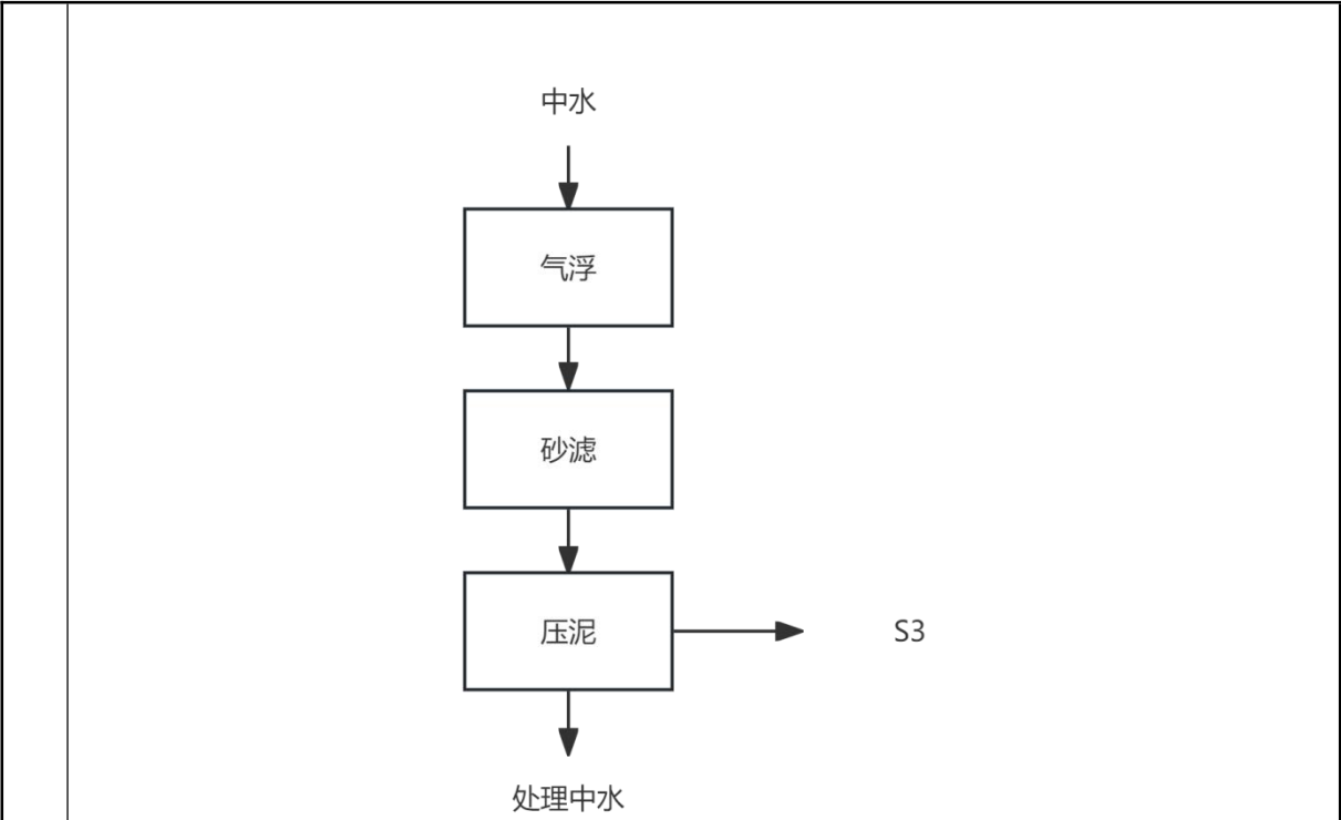
图 2-8 中水处理工艺流程及产污环节示意图
