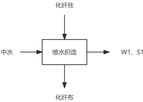
图 2-10 现有项目生产及产污环节示意图
