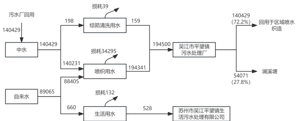
图2-4技改后水平衡图 t/a
