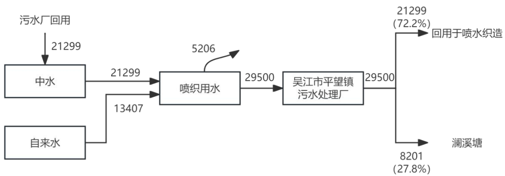
图2-3技改前苏州市潜川纺织有限公司水平衡图 t/a
