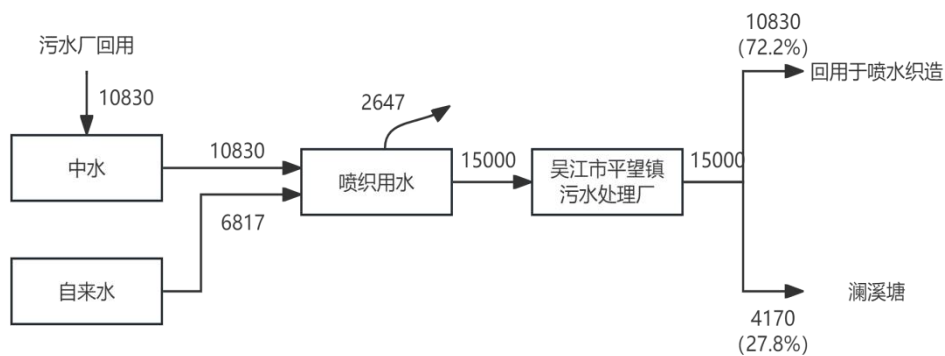
图2-2技改前苏州方润纺织有限公司水平衡图 t/a
