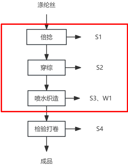
图 2-5 生产工艺流程及产污环节示意图
