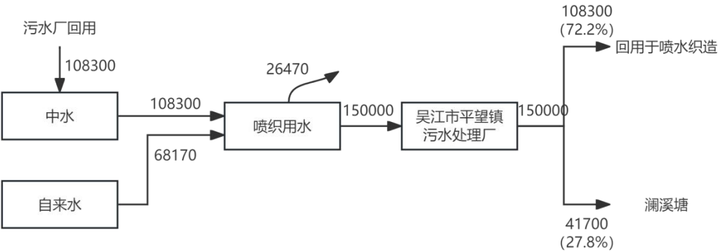
图2-1技改前吴江市伟源纺织品有限公司水平衡图 t/a
