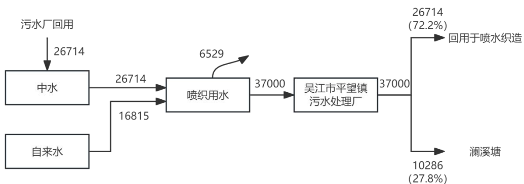
图2-3技改前吴江诚鑫织造有限公司水平衡图 t/a
