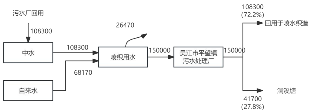
图2-2技改前吴江市金辉丝绸喷织厂水平衡图 t/a
