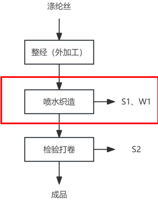
图 2-7 生产工艺流程及产污环节示意图
