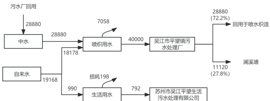
图2-1技改前吴江市振海纺织品有限公司水平衡图 t/a
