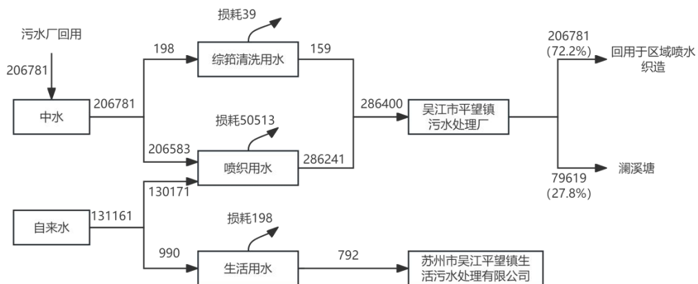
图2-6技改后水平衡图 t/a
