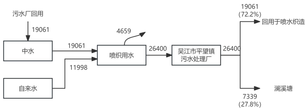
图2-5技改前苏州月与海纺织科技有限公司水平衡图 t/a
