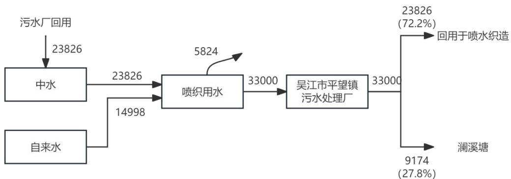
图2-4技改前吴江市业昕织造有限公司水平衡图 t/a
