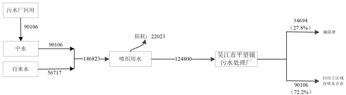
图2-3技改前吴江市兴隆织造有限公司水平衡图 t/a
