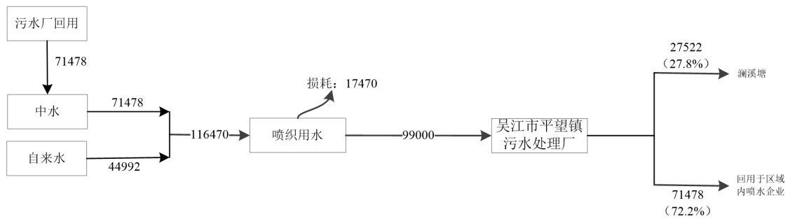
图2-2技改前吴江市雪峰纺织有限公司水平衡图 t/a
