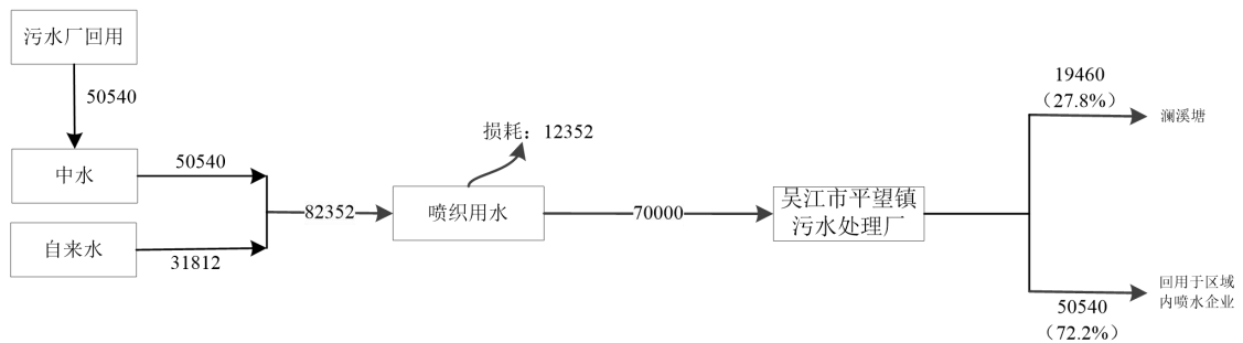
图2-4技改前吴江市振姮织造有限公司水平衡图 t/a
