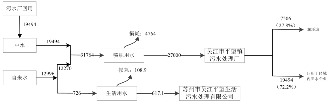
图2-1技改前吴江鑫如织造有限公司水平衡图 t/a
