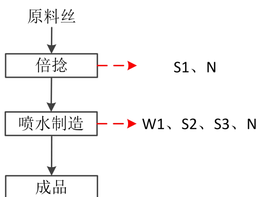
图 2-10 现有项目生产及产污环节示意图
