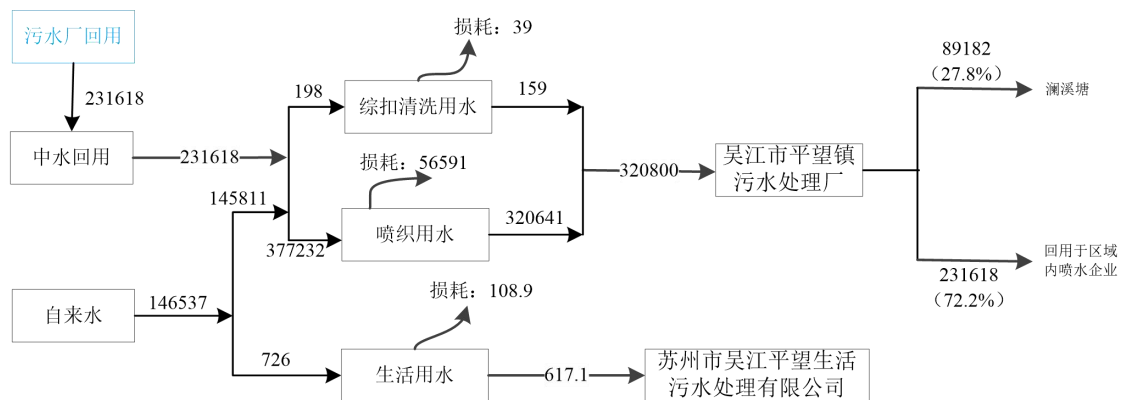
图2-5技改后水平衡图 t/a
