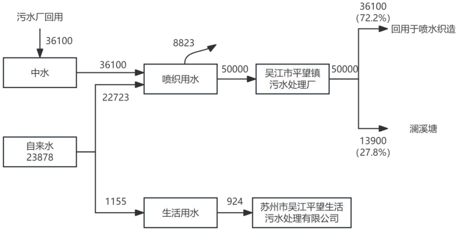
图2-1技改前吴江振洁纺织有限公司水平衡图 t/a
