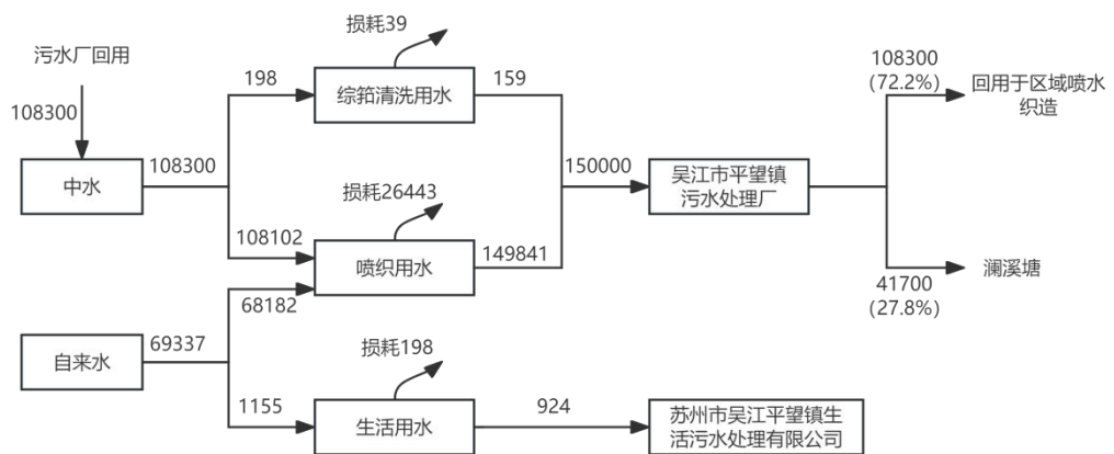
图2-3技改后水平衡图 t/a
