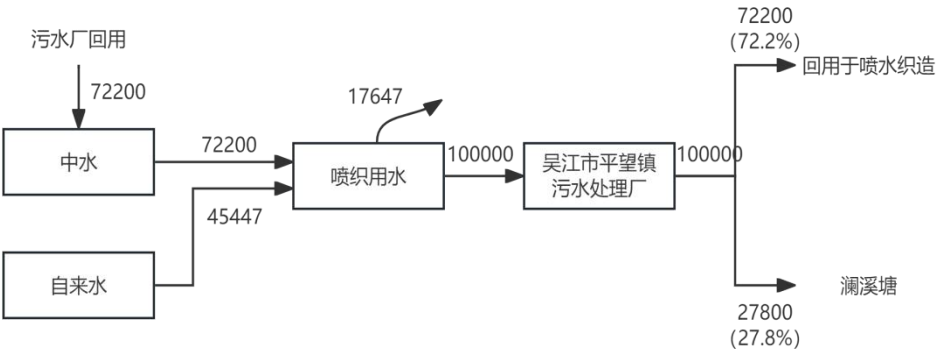
图2-2技改前吴江迎翔织造有限公司水平衡图 t/a
