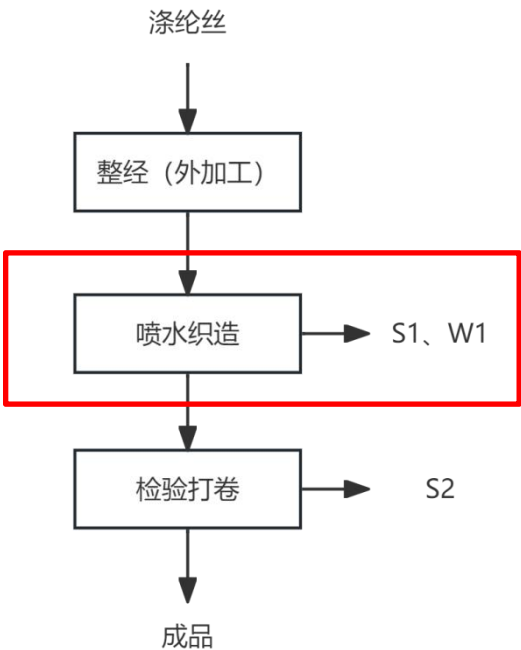
图 2-4 生产工艺流程及产污环节示意图
