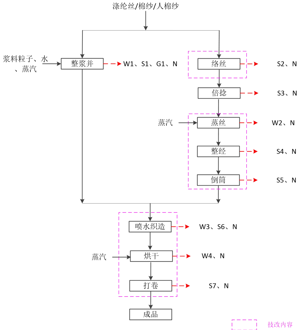
图 2-4 生产工艺流程及产污环节示意图
