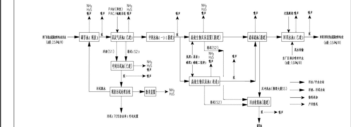
图 4-1 吴江市平望镇污水处理厂处理工艺流程
