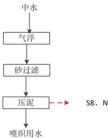
图 2-4 生产工艺流程及产污环节示意图
