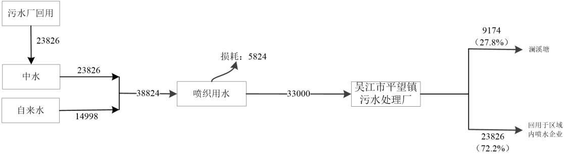
图2-2技改前吴江市新正纺织有限公司水平衡图 t/a
