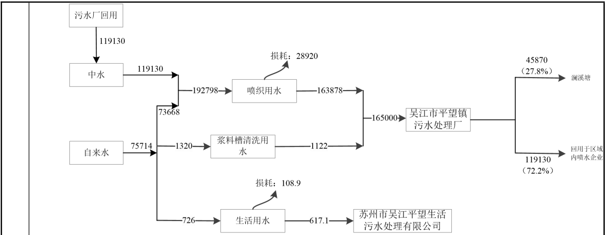
图2-1技改前吴江市新龙强织造有限公司水平衡图 t/a
