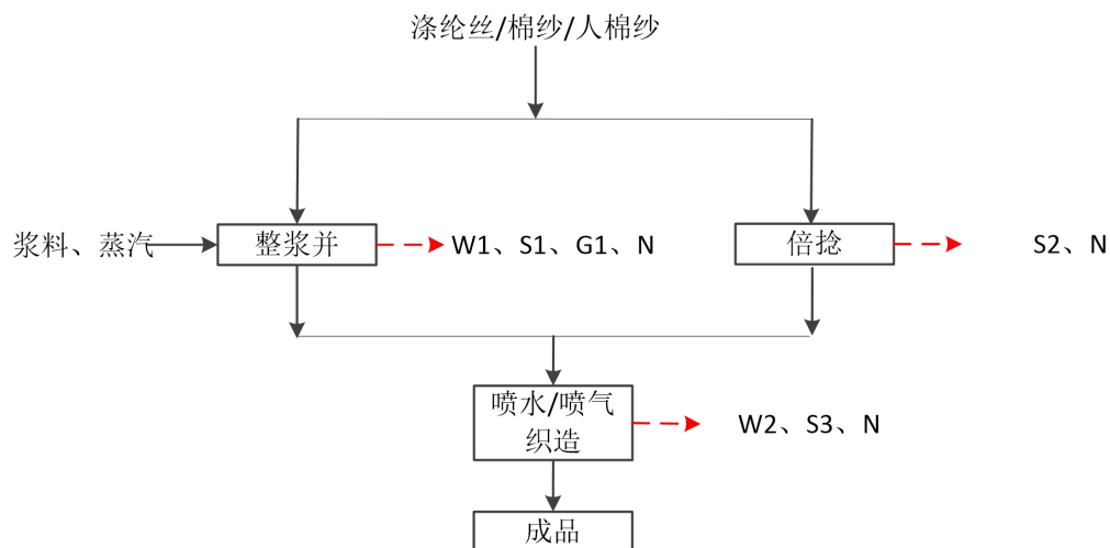
图 2-5 现有项目生产及产污环节示意图
