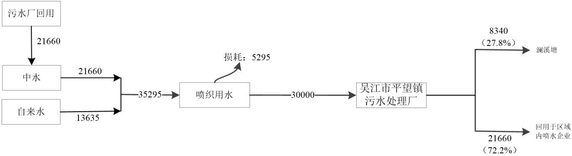
图2-2技改前苏州市璟帝纺织有限公司水平衡图 t/a
