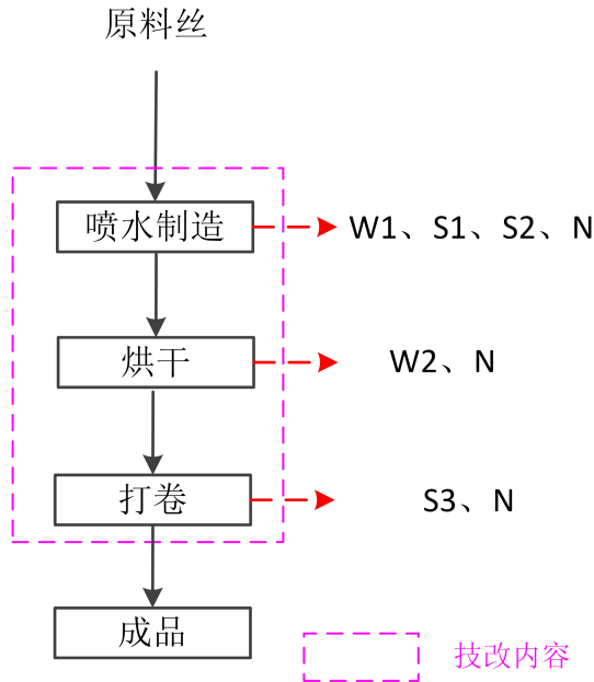
图 2-4 生产工艺流程及产污环节示意图
