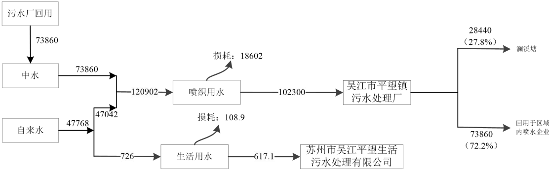
图2-1技改前吴江市平望染料纺织有限公司水平衡图 t/a
