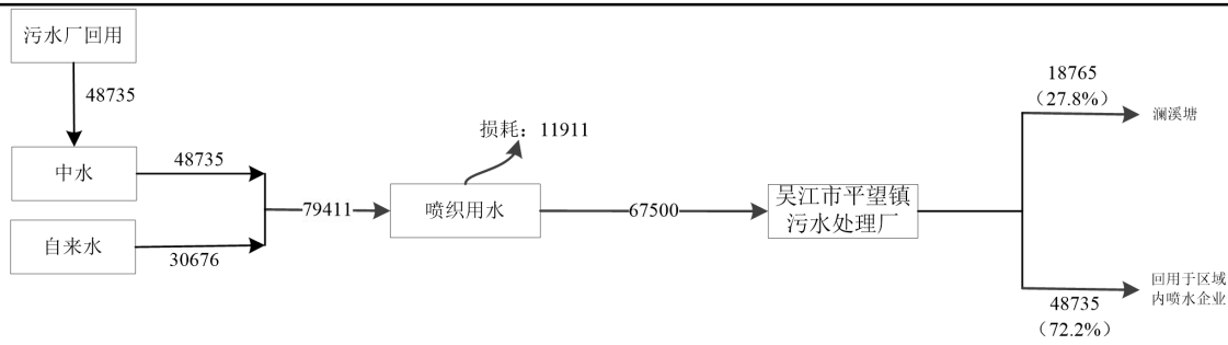
图2-2技改前吴江市世纪同源织造有限公司水平衡图 t/a
