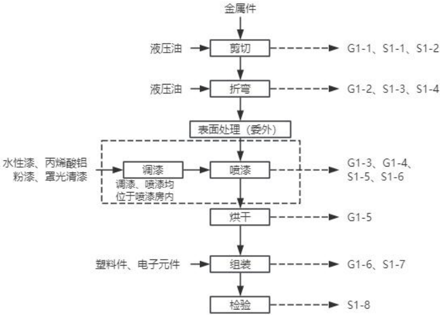
图2-3 汽车配件工艺流程及产污环节示意图
