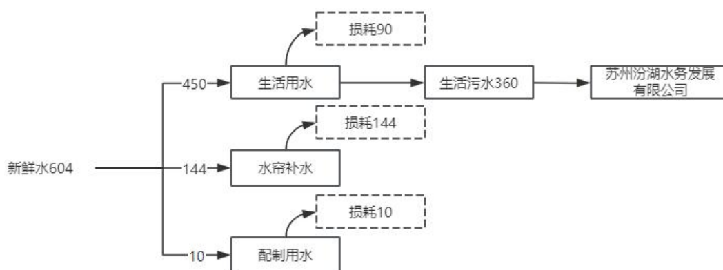
图 2-1 本项目水平衡 t/a
