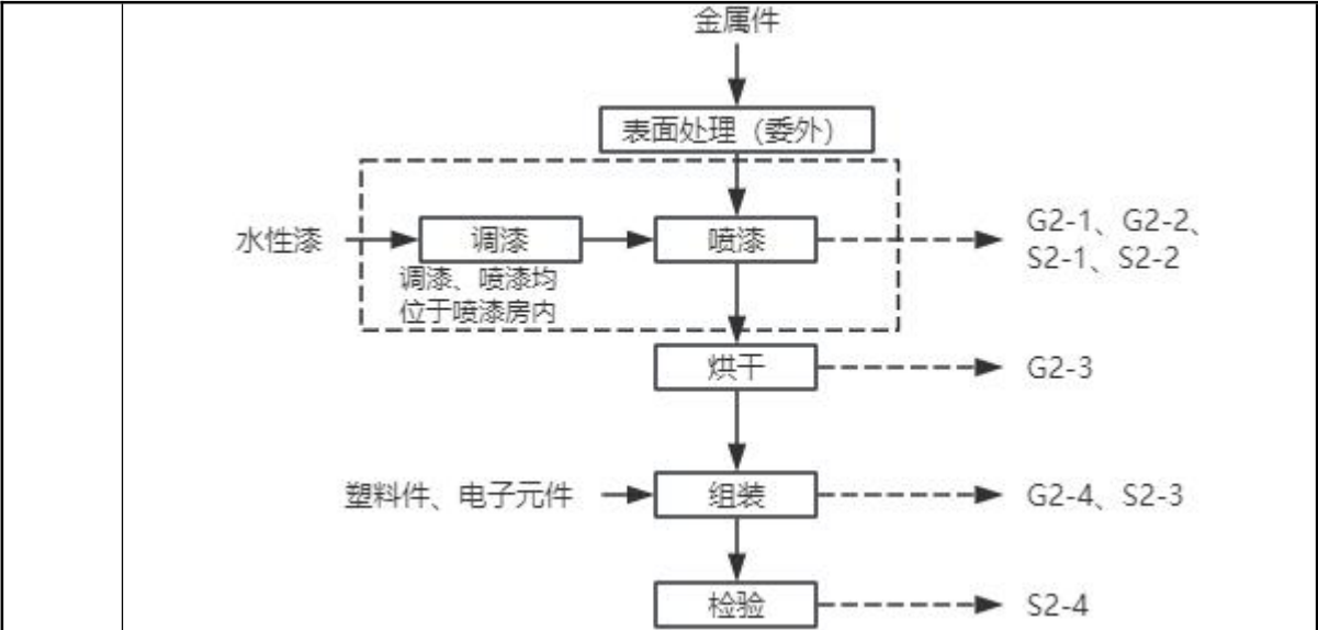
图2-4 电脑配件工艺流程及产污环节示意图
