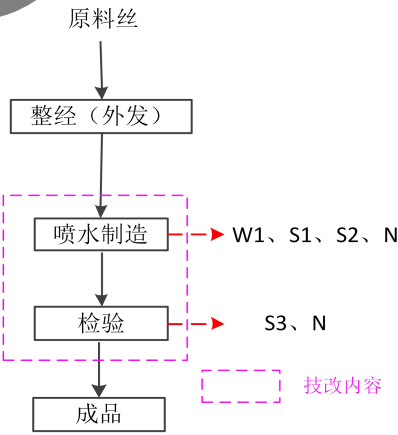
图 2-3 生产工艺流程及产污环节示意图
