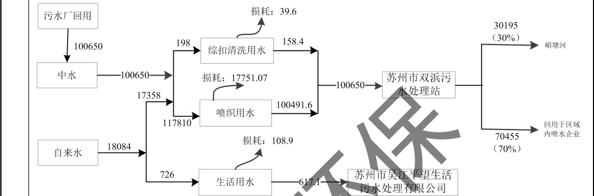
图2-2技改后水平衡图 t/a
