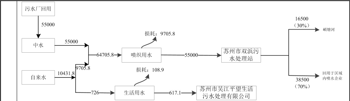
图2-1技改前水平衡图 t/a
