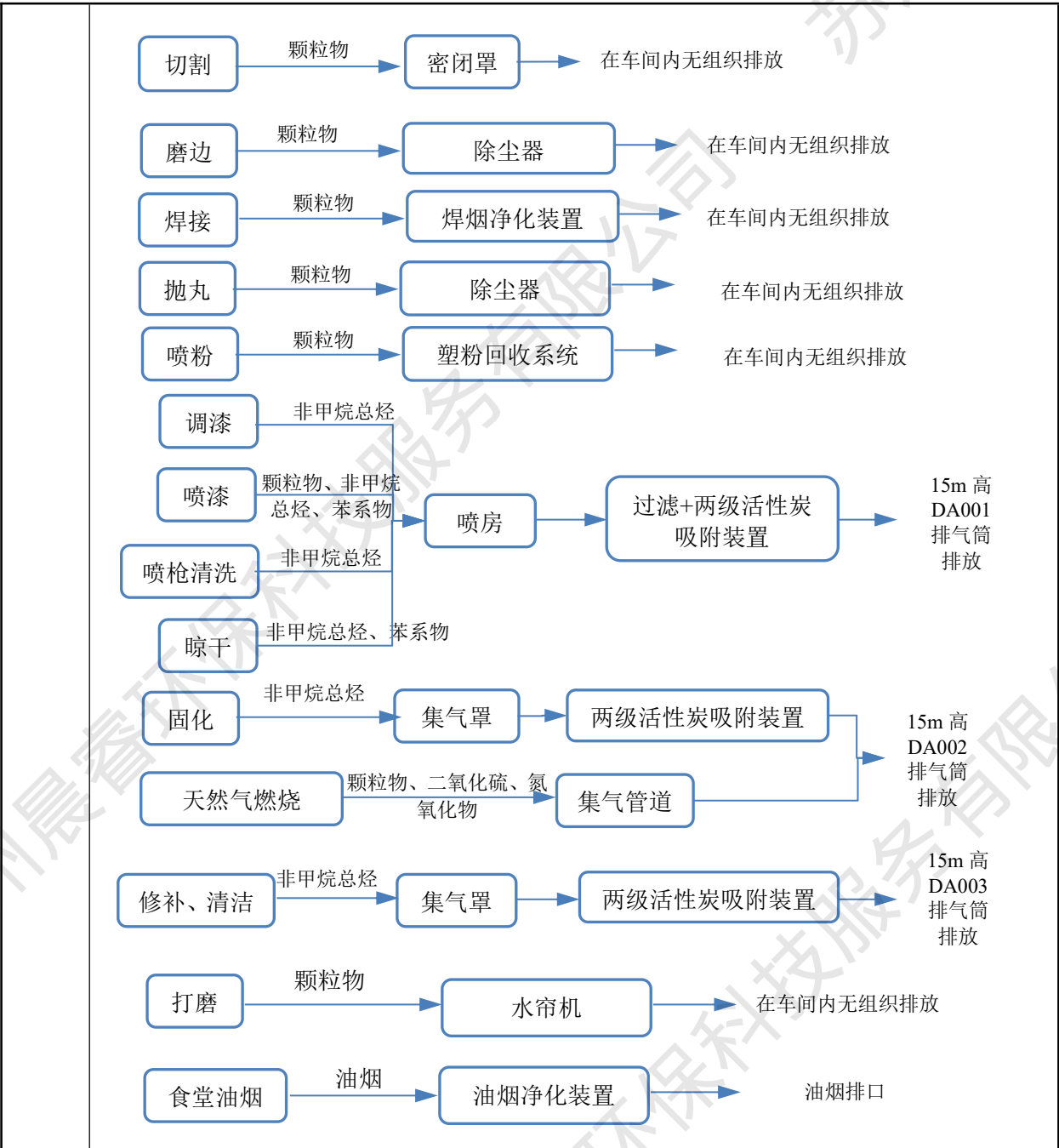
图 4-1 本项目废气收集及处理方式图
