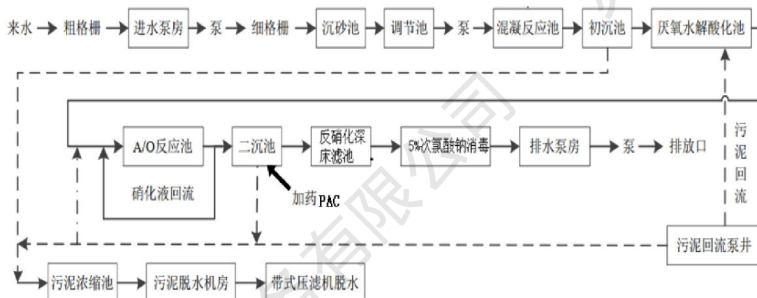
图 4-2 苏州汾湖水务发展有限公司（汾湖城区水质净化厂）工艺流程图
