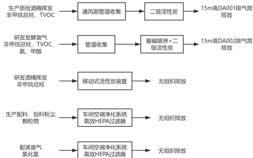
图 4-2 废气收集图
