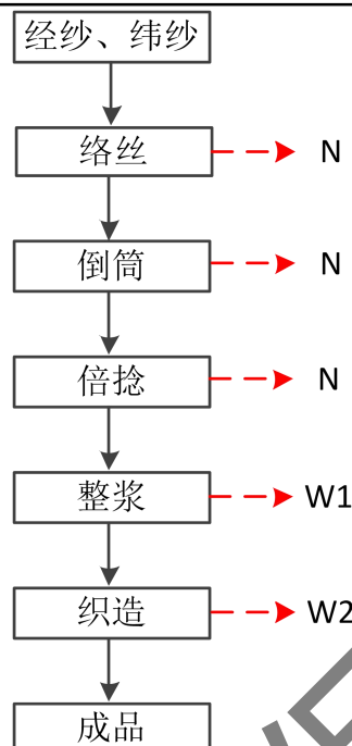
图 2-3 现有项目生产及产污环节示意图
