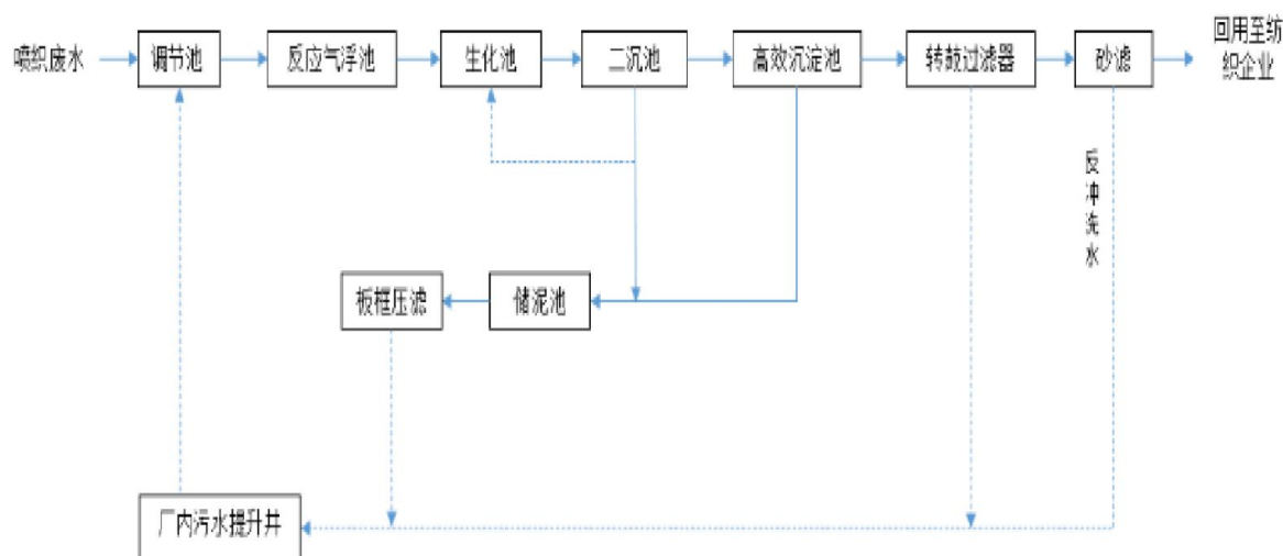
图 4-1 盛泽镇南麻社区综合污水处理厂（工业）喷织废水处理工艺流程
