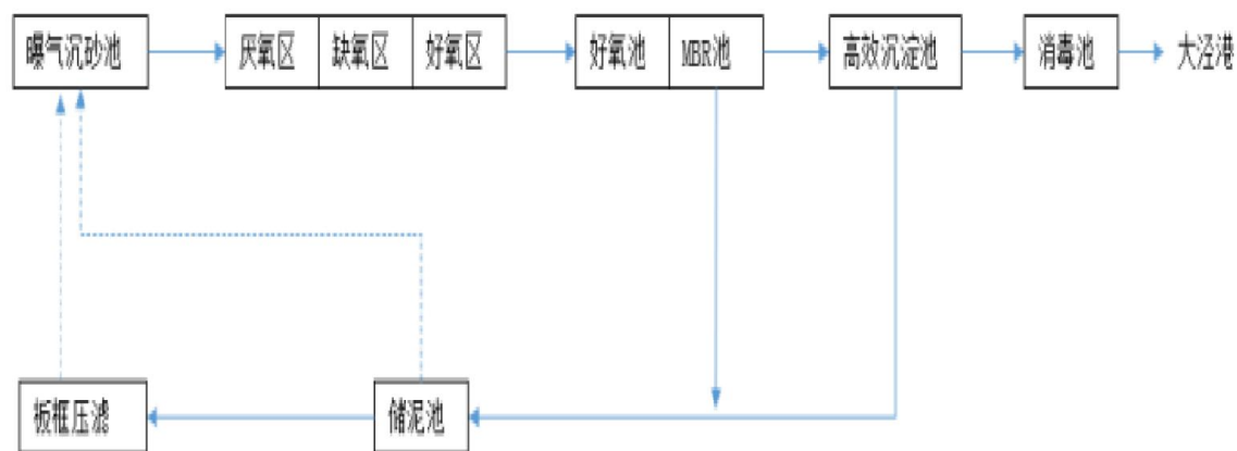
图 4-2 盛泽镇南麻社区综合污水处理厂（生活）生活污水处理工艺图
