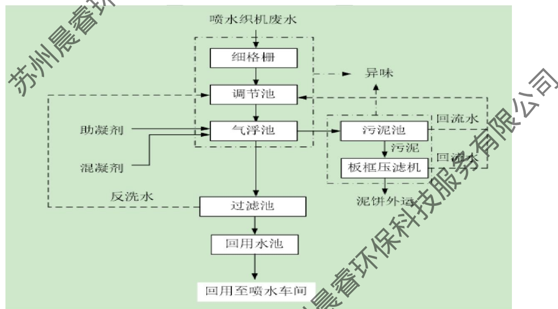
图 4-1 吴江市平望污水处理厂处理工艺流程
