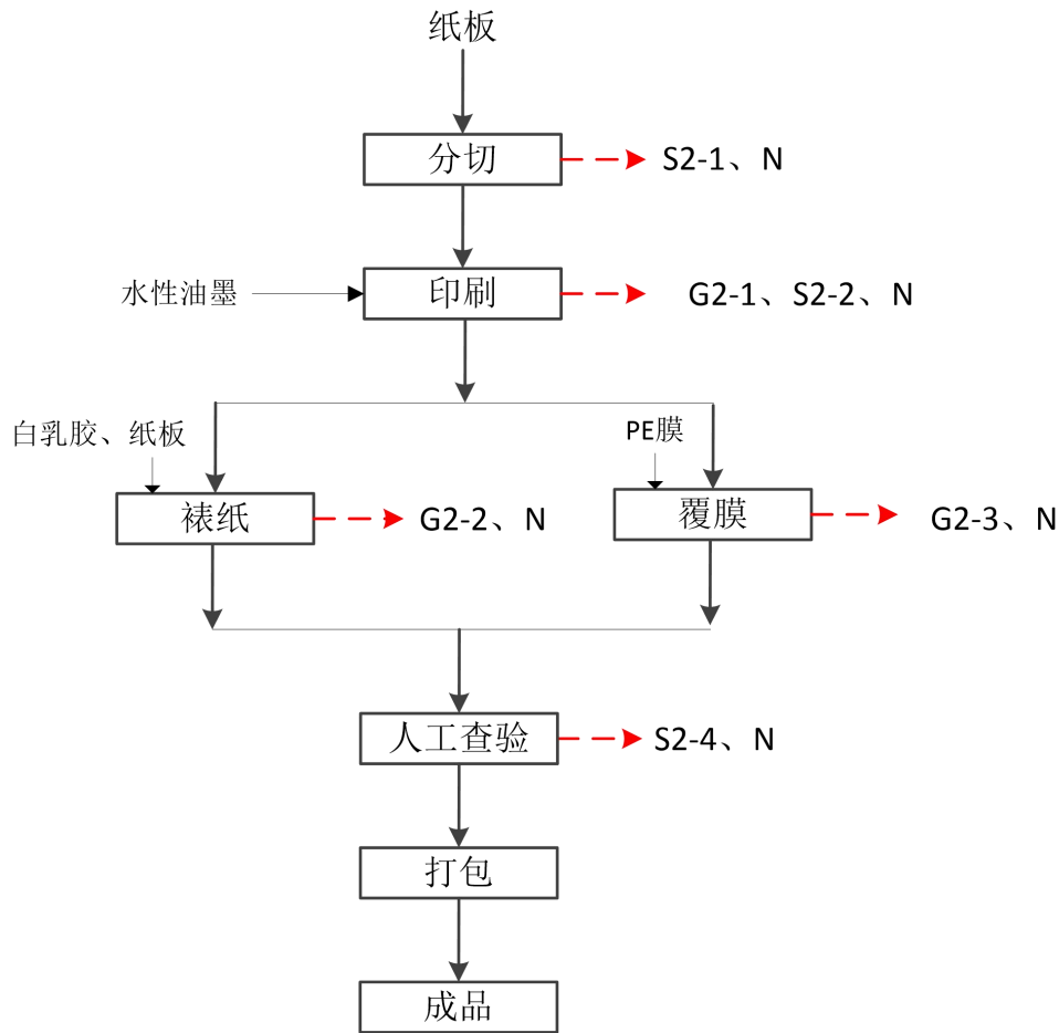
图 2-3 纸板生产工艺流程
